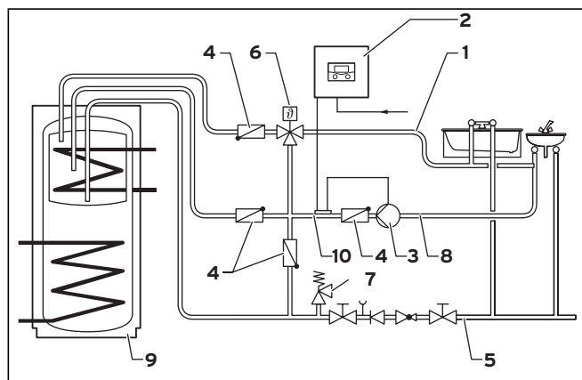
Рис. 6.4 Термостатический смеситель горячей воды в циркуляционной линии
