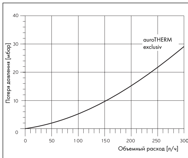
Рис. 8.4 Потеря давления коллектора auroTHERM exclusiv
