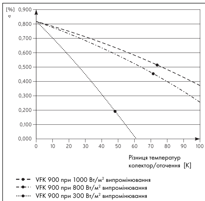
Мал. 8.7 ККД відповідно до DIN EN 12975
