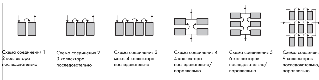
Рис. 11.4 Схемы соединений плоских коллекторов autoTHERM от Vaillant (макс. 4 последовательно)
