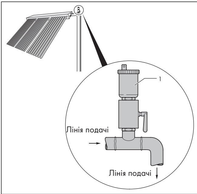
мал. 6.1 Швидкодіючий збеповірювач геліоустановки
