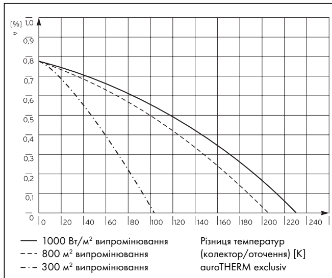
Мал. 8.3 ККД відповідно до DIN EN 12975 auroTHERM exclusiv
