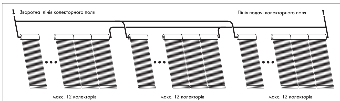
Мал. 11.3 Схема сполучень більше, ніж для 12 трубчатих сонячних колекторів autoTHERM exclusiv разом з послідовним та паралельним підключенням
