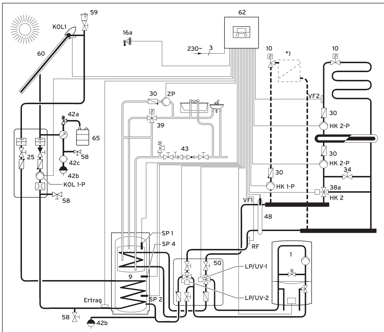
Мал. 3.2 Геліосистема для підтримки опалення та підігріву питної води комбінованим водонагрівачем auroSTOR регульованою інтеграцією системи опалення (гідралічний блок) та газовим насти́ним опалювальний пристроєм.
