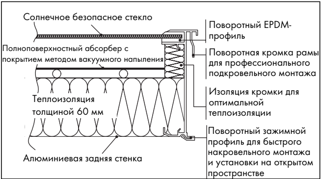
Рис. 8.6 Плоский коллектор auroTHERM от Vaillant в разрезе
