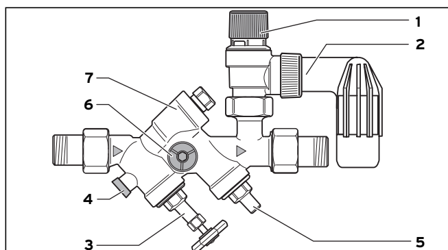
Рис. 4.3 Установка групп безопасности
