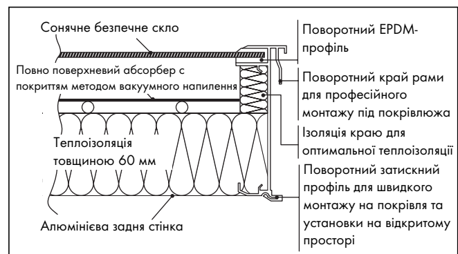
Мал. 8.6 Розріз плоского коллектора auroTHERM
