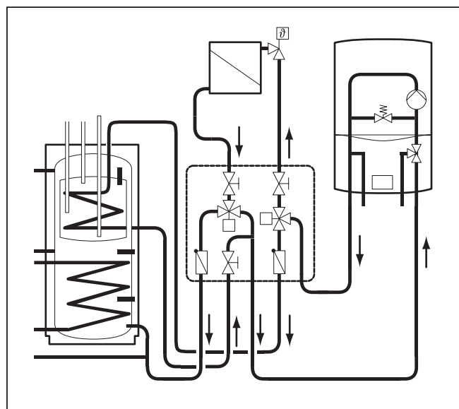
Рис. 5.2 Интеграция гидравлического блока
