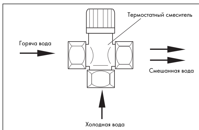
Рис. 6.3 Термостатический смеситель горячей воды
