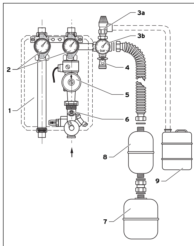
Рис. 7.1 Конструкция насосной группы гелиоустановки 6 л/мин либо 22 л/мин
