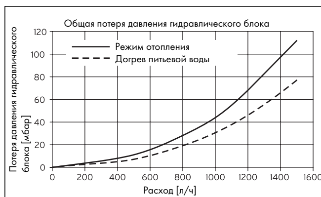
Рис. 5.3 Потеря давления гидравлического блока
