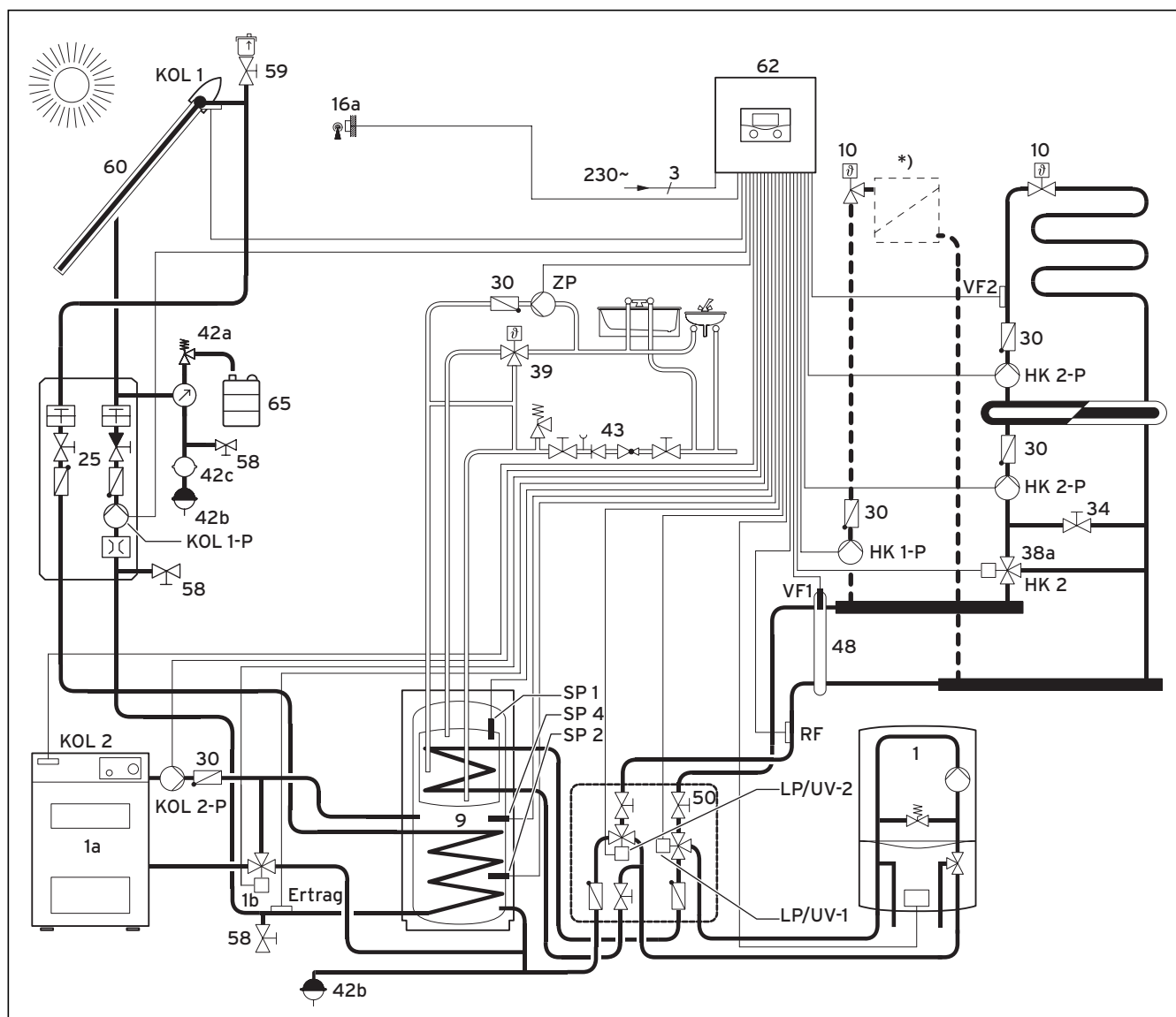
Мал. 3.3 Геліосистема для підтримки опалення та підігріву питної води комбінованим водонагрівачем auroSTOR регульованою інтеграцією системи опалення (гідралічний блок) та котлом, який працює на твердому паливі.
